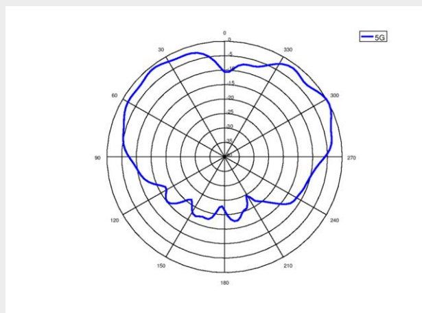
5G-2 (PHI=90)
