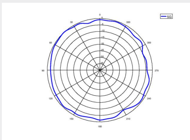
5G-2 (PHI=0)
