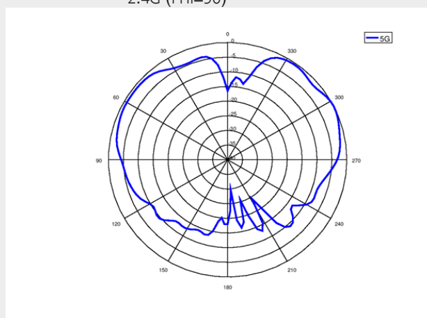
5G-1 (PHI=90)
