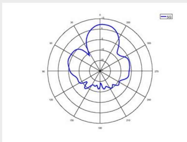
5G (PHI=90)
